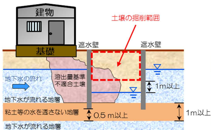
粘土等の水を透さない地層より 浅い地層を掘削する場合
