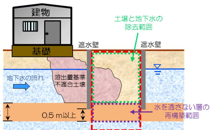
粘土等の水を透さない地層より 深い地層を掘削する場合
